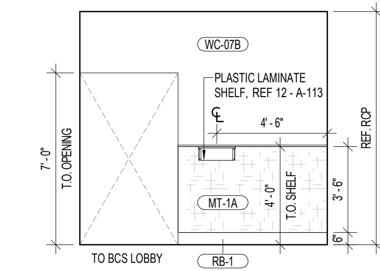
5 MESSAGE 1/4" = 1'-0"
