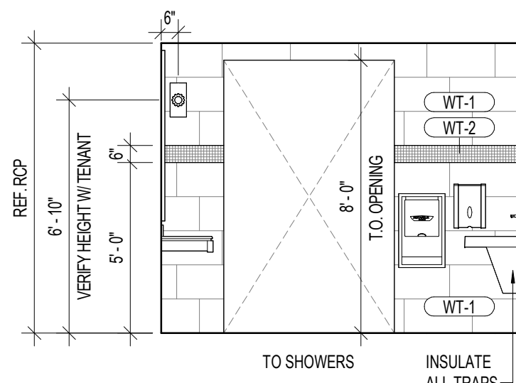
9 VANITIES (S.O.H.) 1/4" = 1'-0"
