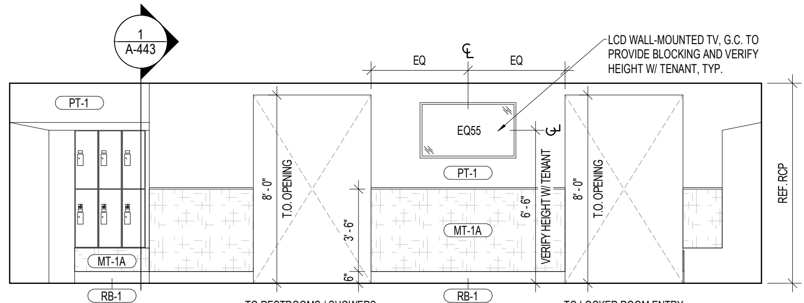
7 LOCKER ROOM (S.O.H.) 1/4" = 1'-0"
