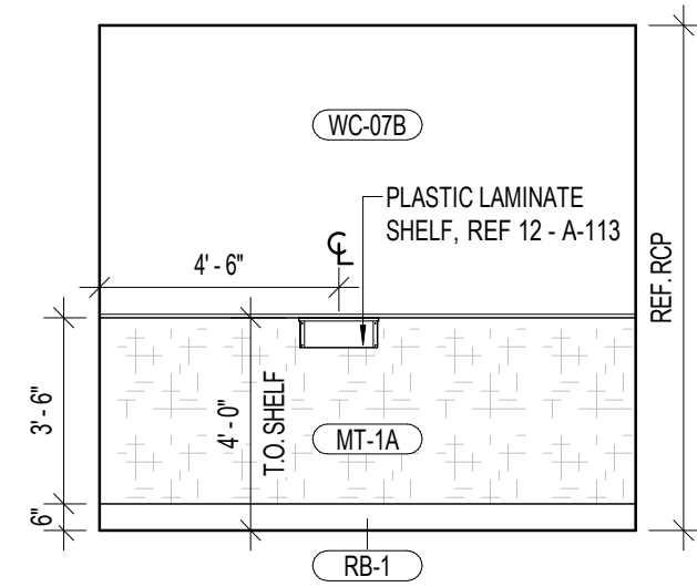
7 MESSAGE 1/4" = 1'-0"
