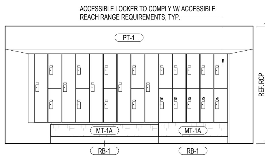
6 LOCKER ROOM (S.O.H.) 1/4" = 1'-0"
