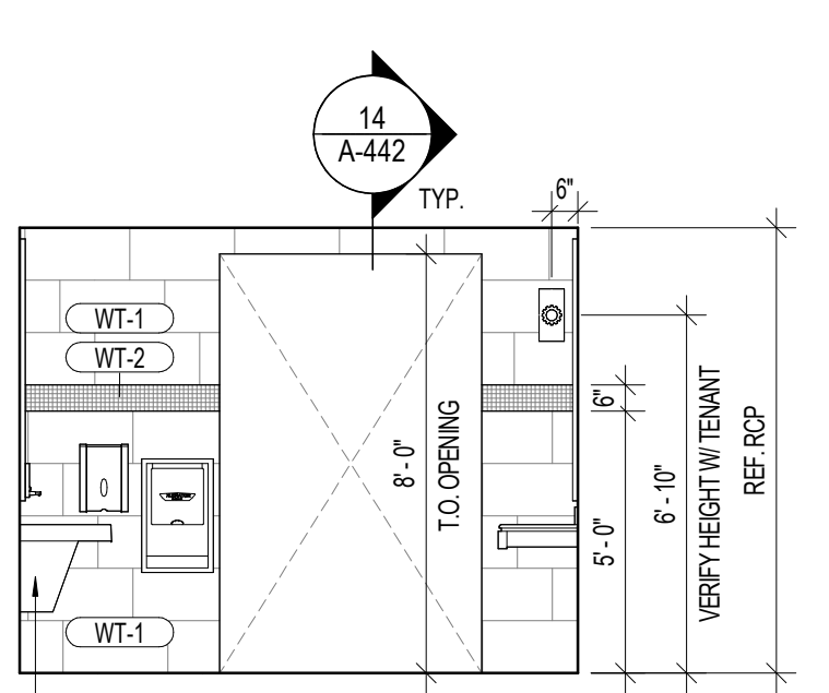
11 VANITIES (S.O.H.) 1/4" = 1'-0"
