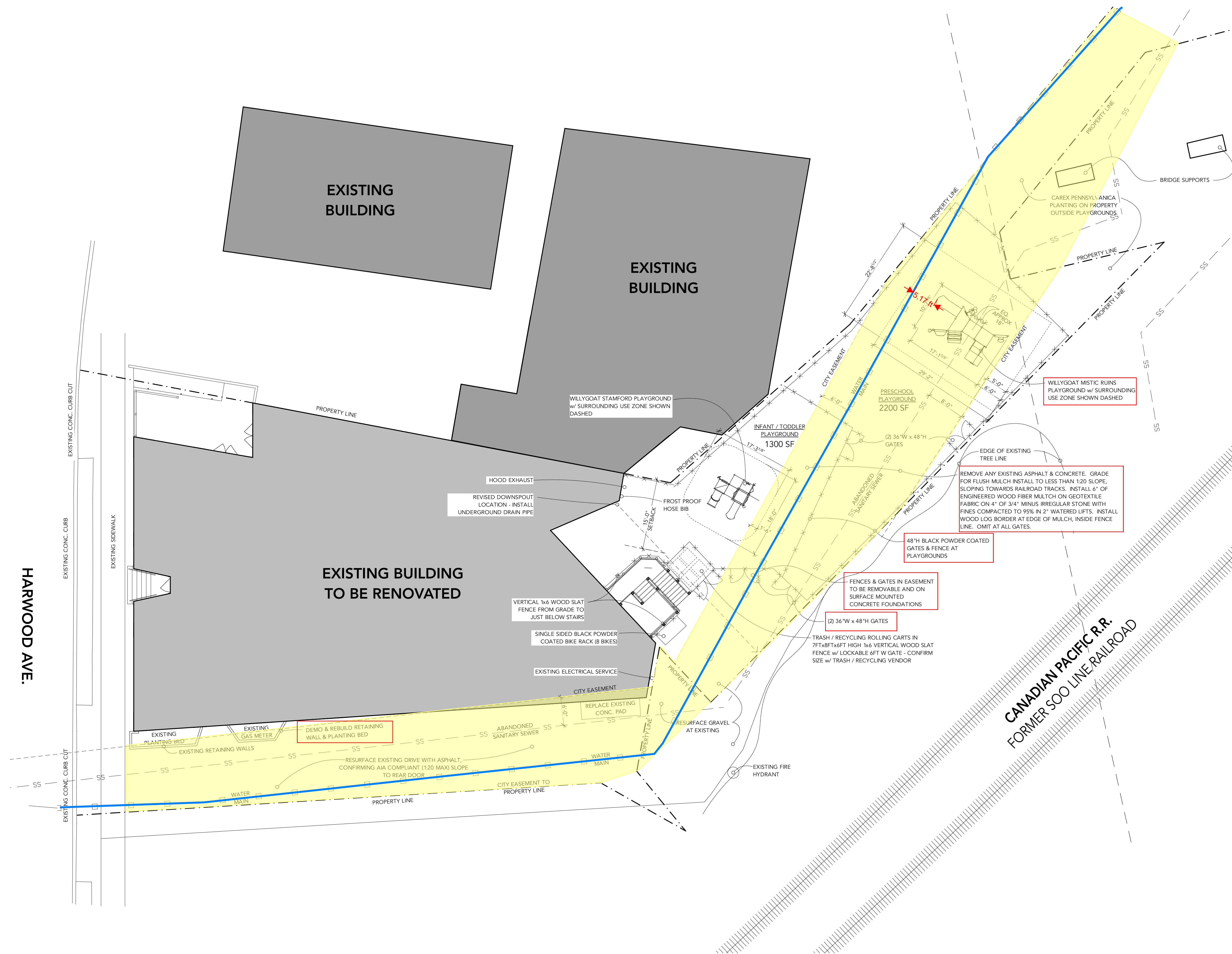
1 Site Plan SCALE: 1" = 10'
